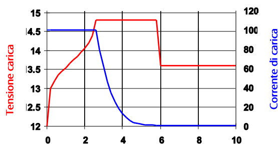
Fig. 3: Curva di carica in 3 fasi
